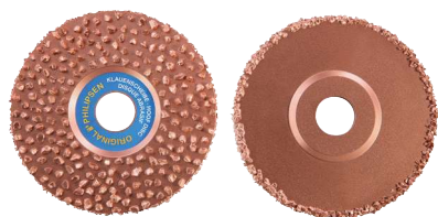
DISCO ABRASIVO PER ZOCCOLI "PHILIPSEN" DUE LATI (GRANA 30 ANT. - 10 POST.) Ø 115 MM
