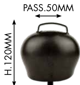
SONNAILLE POUR BOVINS "CAPRIOLO" (TYPE PREMANA) FAITE À LA MAIN EN ACIER BOMBÉ N°9 (H.120 MM - PASS.50 MM)
