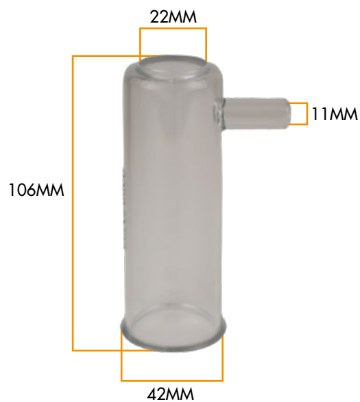
BOSSOLO IN PLASTICA PER GUAINA MUNGITURA OVINI 04.04.0406
