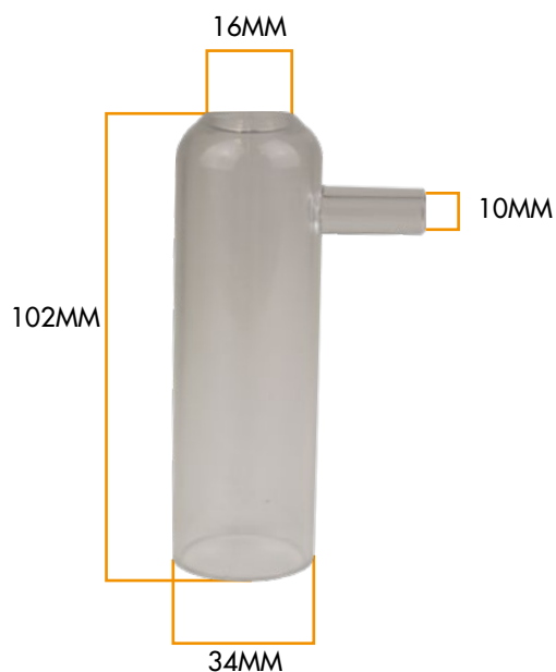
BOSSOLO IN PLASTICA PER GUAINA MUNGITURA OVINI 04.04.0402
