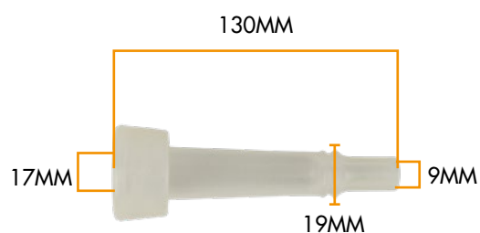
GUAINA IN SILICONE PER MUNGITURA OVINI
