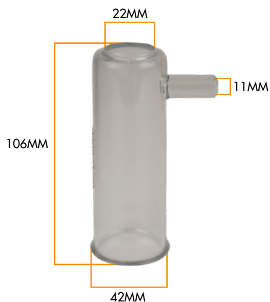
GOBELET EN PLASTIQUE POUR LA TRAITE DES OVINS 04.04.0406
