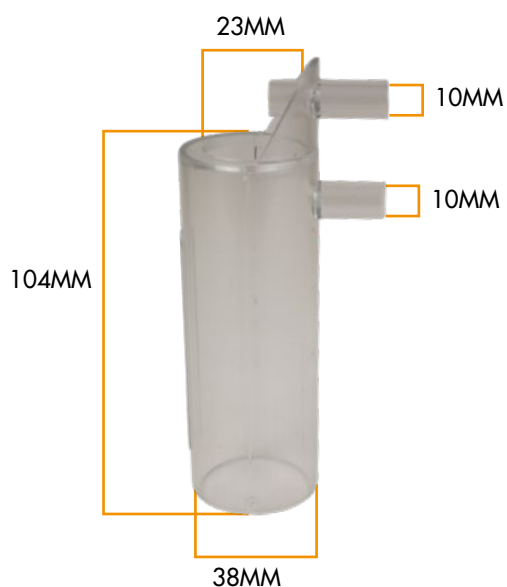
GOBELET EN PLASTIQUE POUR LA TRAITE DES OVINS 04.04.0404
