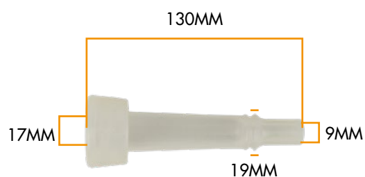
MANCHON EN SILICONE POUR LA TRAITE DES OVINS
